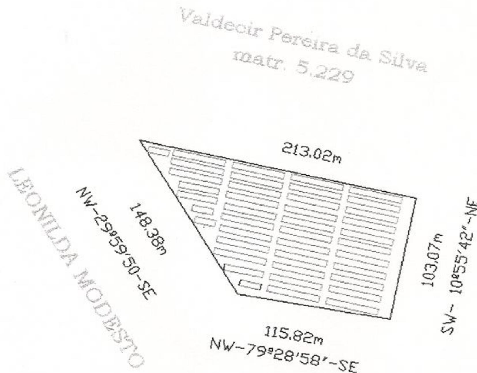
Figura 07 - Mapa demonstrativo sem escala, dimensionamento das valas do Aterro Municipal.
